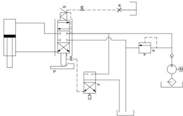
结构原理图
